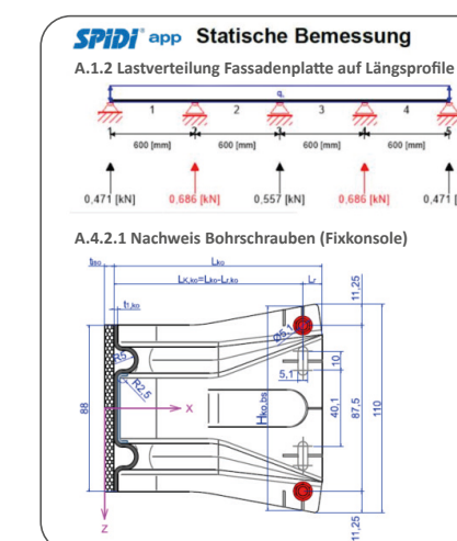
Beispiel Statik
