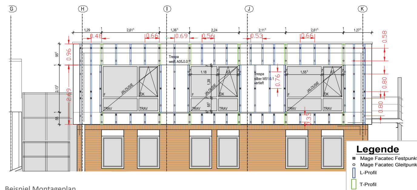
Beispiel Montageplan
